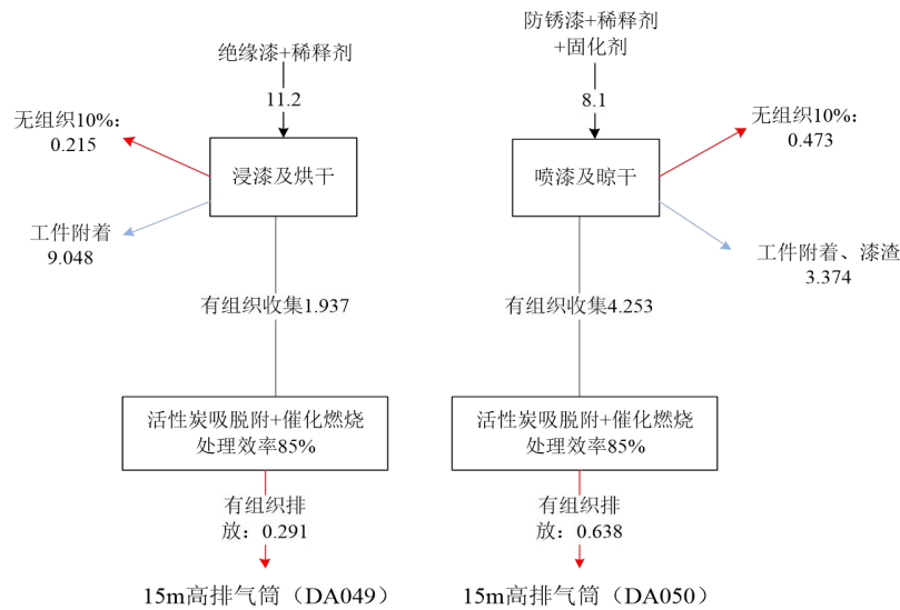
图 3.2-6 含 VOCs 物料平衡图
