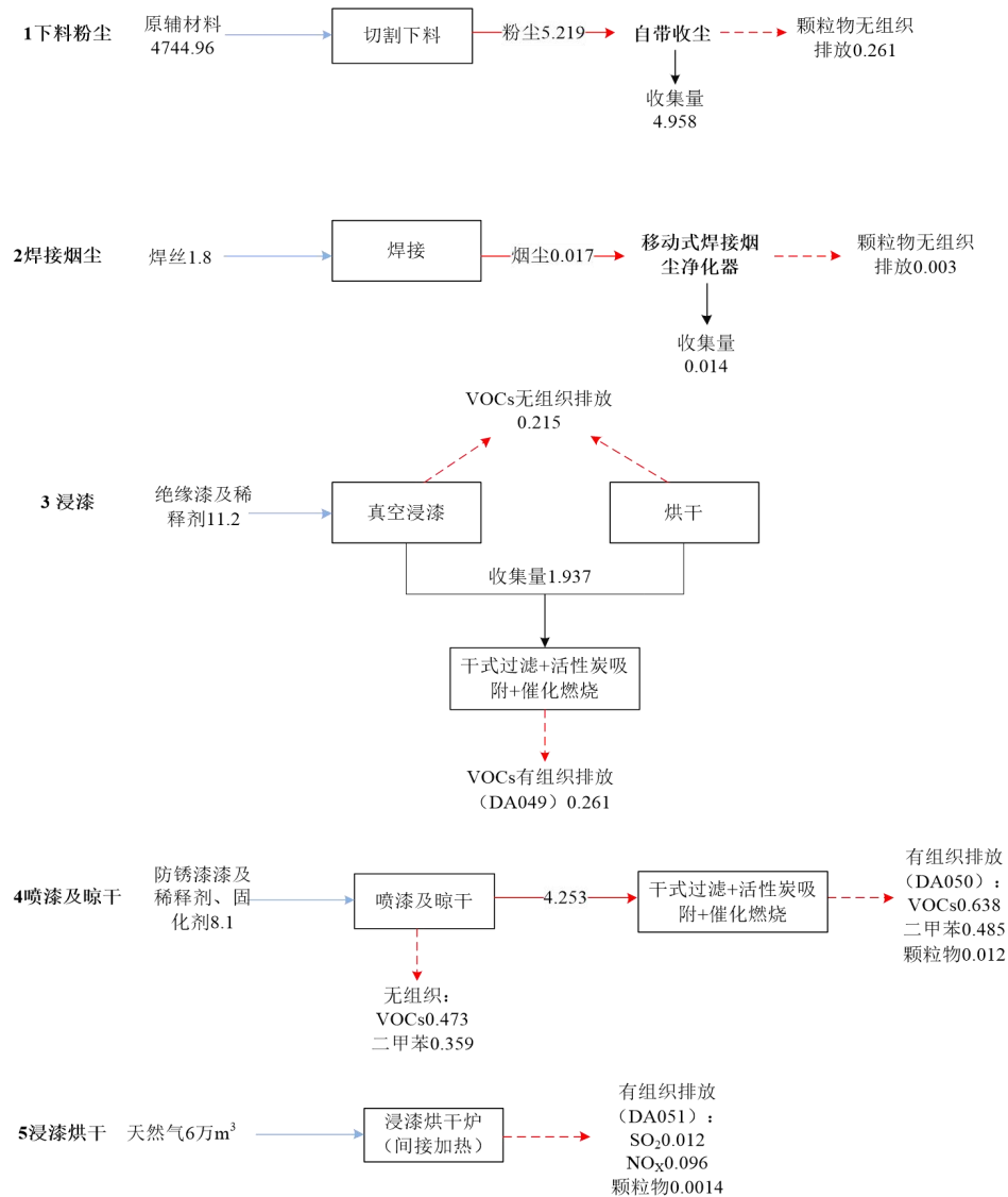
图 3.2-7 运营期废气产生及排放走向情况
