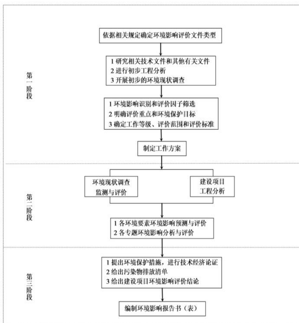
图2 评价工作流程图
