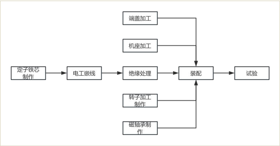
图 3.2-1 运营期总体生产工艺流程图
