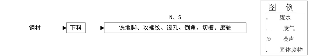
图 3.2-5 转轴及转子程及排污节点
