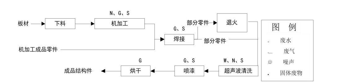
图 3.2-4 组件机加工工艺流程及排污节点
